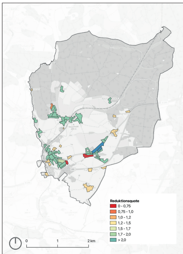
Abb. 15: Reduktionsquoten in den Versorgungsgebieten (%)
