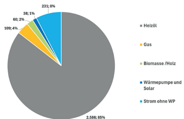
Abb. 9: Treibhausgasemissionen nach Energieträger (t/a)
