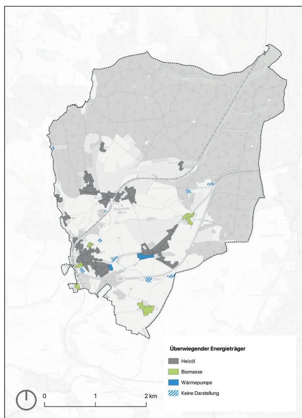
Abb. 5: Überwiegender Energieträger
