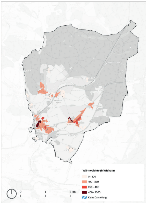
Abb. 3: Wärmedichte (MWh pro Hektar und Jahr)
