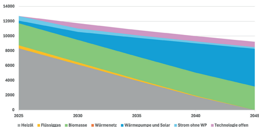
Abb. 18: Zielszenario: Prognose Wärmebedarf nach Energieträger (MWh/a)
