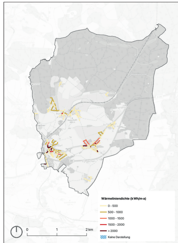
Abb. 4: Wärmelinien-dichte (kWh pro Meter und Jahr)
