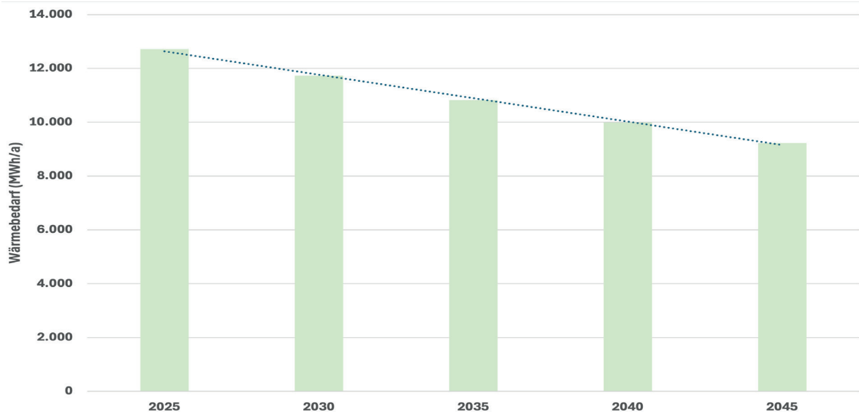
Abb. 14: Entwicklung des zukünftigen Wärmebedarfs bis 2045
