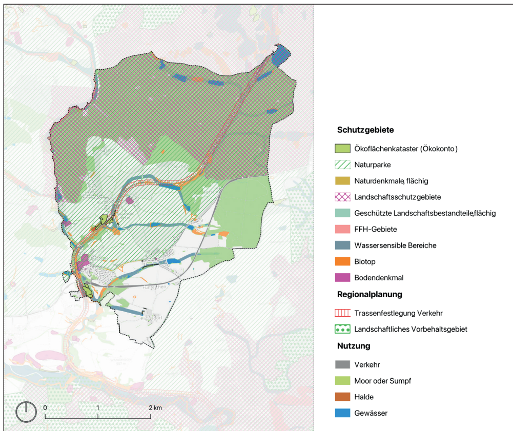
Abb. 11: Flächenscreening
