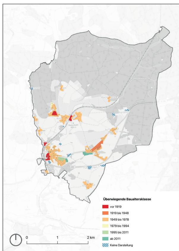
Abb. 7: Überwiegende Baualtersklasse
