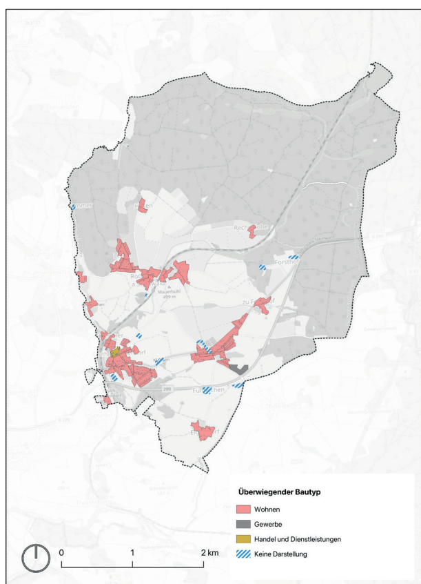
Abb. 6: Überwiegender Bautyp
