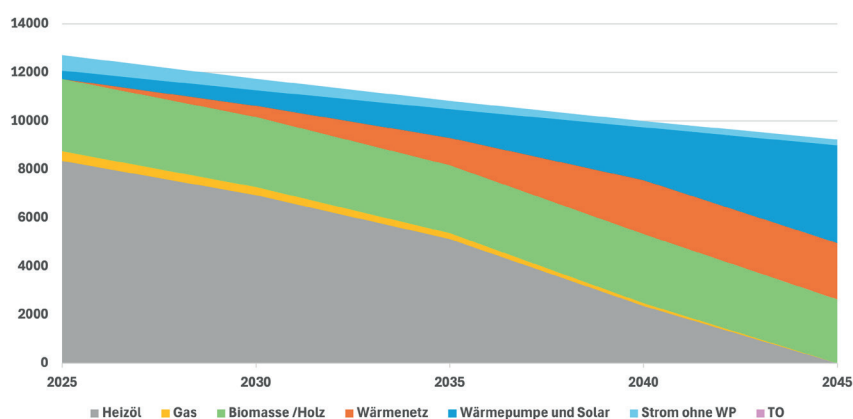
Abb. 16: Szenario „Maximaler Wärmenetz-Ausbau“: Prognose Wärmebedarf nach Energieträger (MWh/a)
