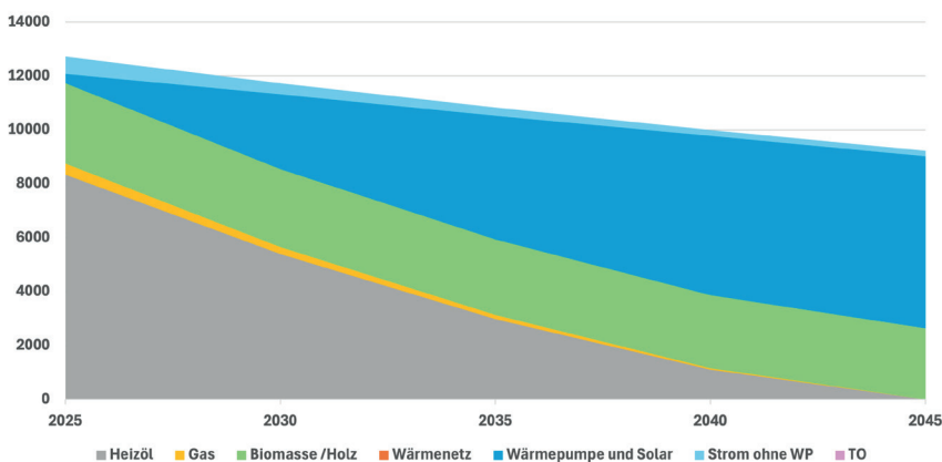
Abb. 17: Szenario „Maximaler Wärmepumpen-Ausbau“: Prognose Wärmebedarf nach Energieträger (MWh/a)
